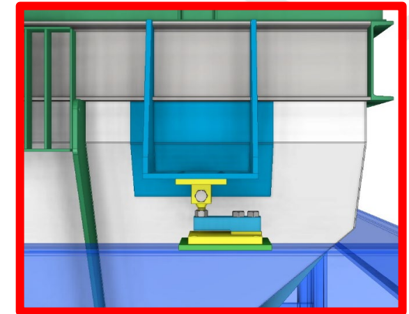
DETALLE CELDAS DE CARGA
